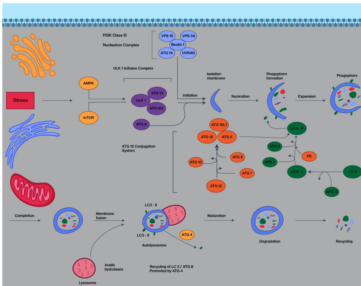
Fig. 1. Autophagy process.
